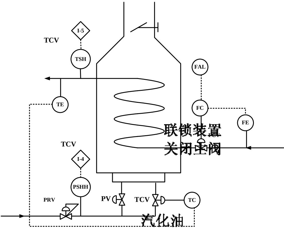
图B. 4 油蒸发器
